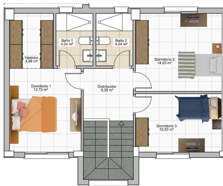
PLANTA PRIMERA
