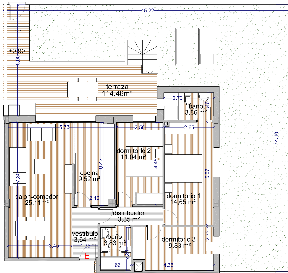
Vivienda_Planta baja
